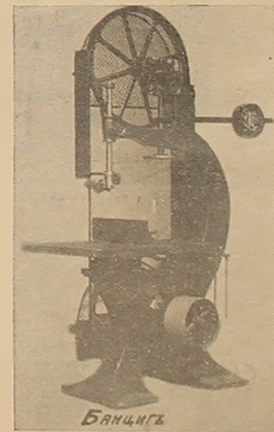
Банцигъ — Производство на Машинна кооператив. ф-ка „Стомана“ — Пловдивъ (текстъ — стр. 18)
