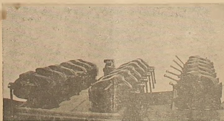
Въртящи паралелни менгемета. — Производство на маш. кооператив. ф-ка „Стомана“ — Пловдивъ (текстъ — стр. 18)
