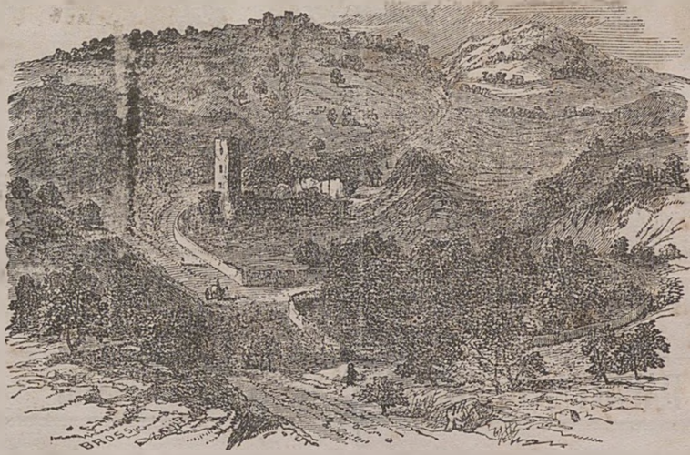
Геосиманія
