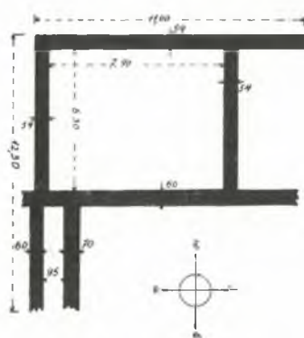
Обр. 198. — Планъ на римската сграда въ Марцианополъ. Fig. 198. — Plan d'une maison romaine à Marcianopolis.
