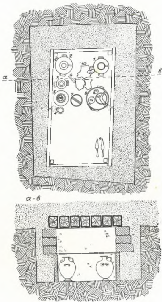
Обр. 6. — Планъ и разрѣзъ на гробницата въ Башова могила.
