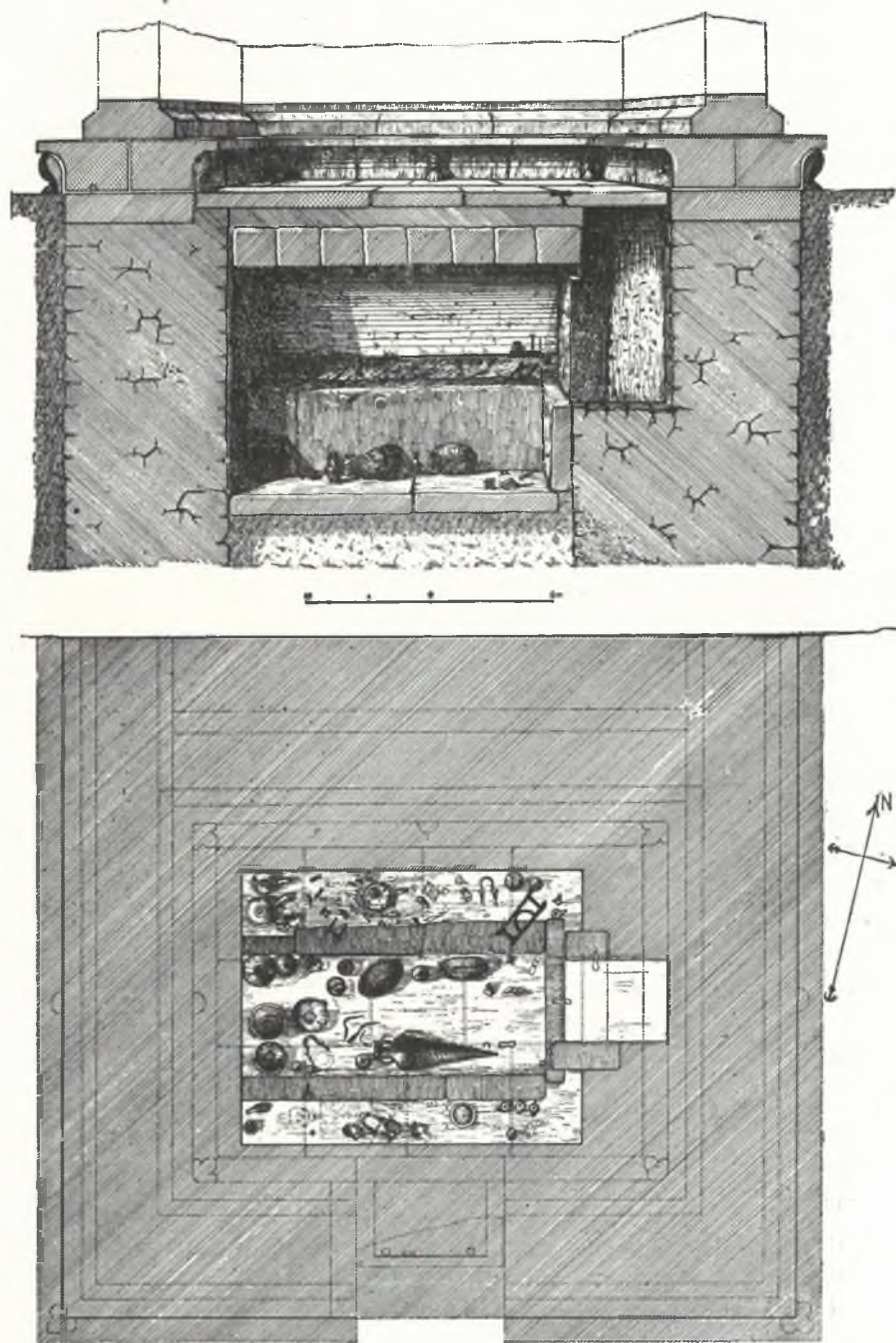
Обр. 41. — Вертикаленъ разрѣзъ и планъ на гробницата отъ Балчикъ. Fig. 41. — Coupe verticale et plan du tombeau de Balčik.
