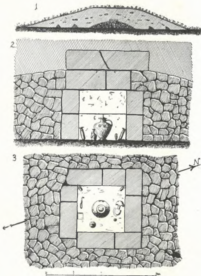
Обр. 50. — Гробницата въ могилата Сезъ-севмесъ при Варна: вертикаленъ разрѣзъ и планъ.
