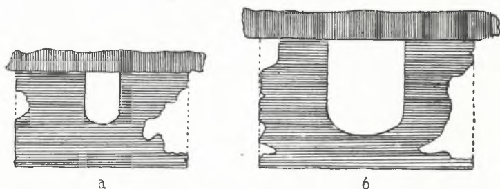
Обр. 200. — Напрѣченъ разрѣзъ на римскитѣ водопроводи на Novae.
