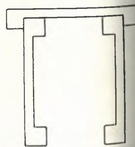
Рис. 28. Перпендикулярный разрез водоотводного канала
