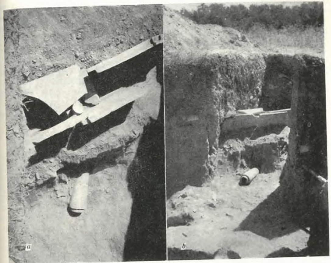
Рис. 29 а. Водоотводный канал и фрагмент глиняного трубопровода. Вид сверху. б. Глиняный трубопровод и канал из черепиц. Сондаж С
