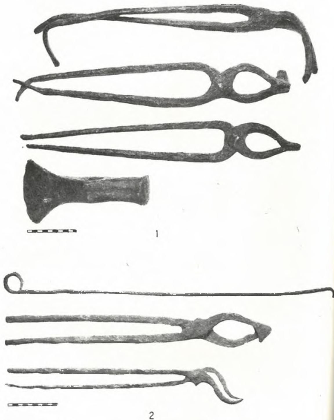
Табл. II. Орѣдия на труда: 1 — с. Смолянци, Михайловградско; 2 — с. Крупник, Благоевградско Pl. II. Outils. 1 — vill. Smolianovci, arr. de Mihailovgrad; 2 — vill. Krupnik, arr. de Blagoevgrad.
