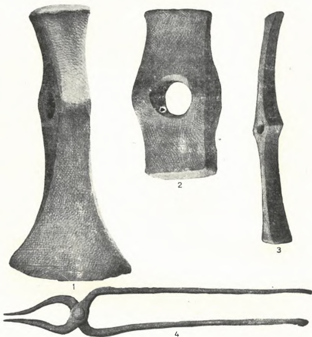
Обр. 12. Ковашки инструменти
