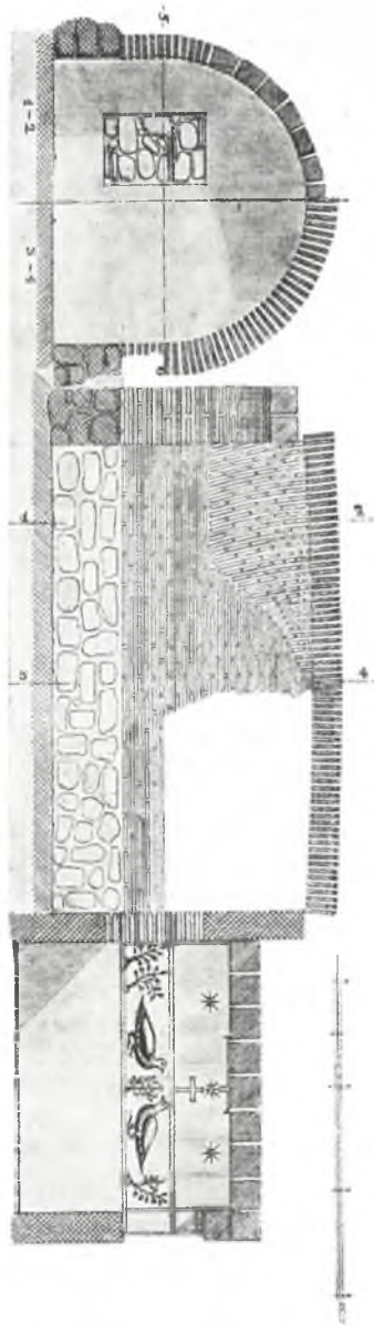
Abb. 336. Разрѣзи презъ старохристиянскитѣ гробници № I и II въ Софин Öbr. 336. Quer- und Längsschnitte durch die altchristlichen Grabkammern № I und II in Sofia
