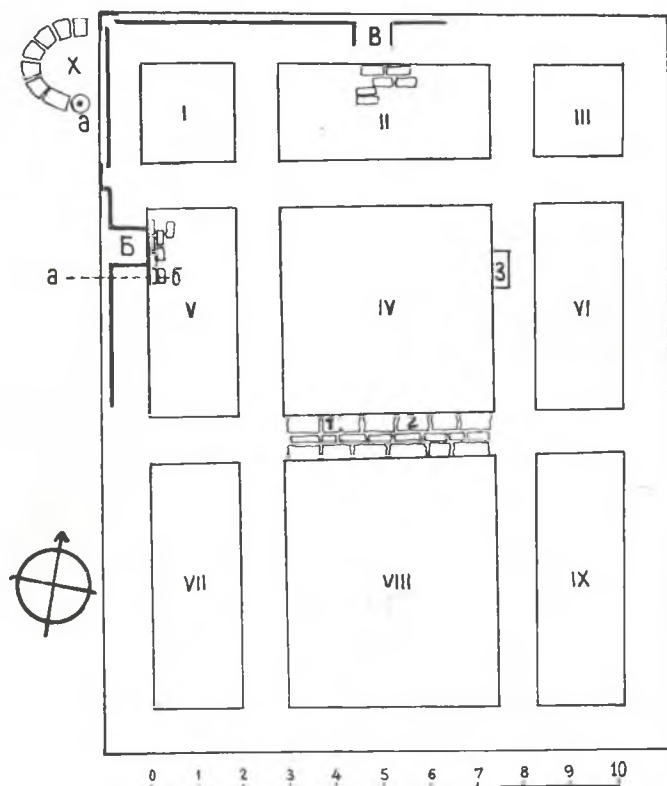
Обр. 158. Планъ на болярското жилище Abb. 158. Grundriss der Boljarenwohnung
