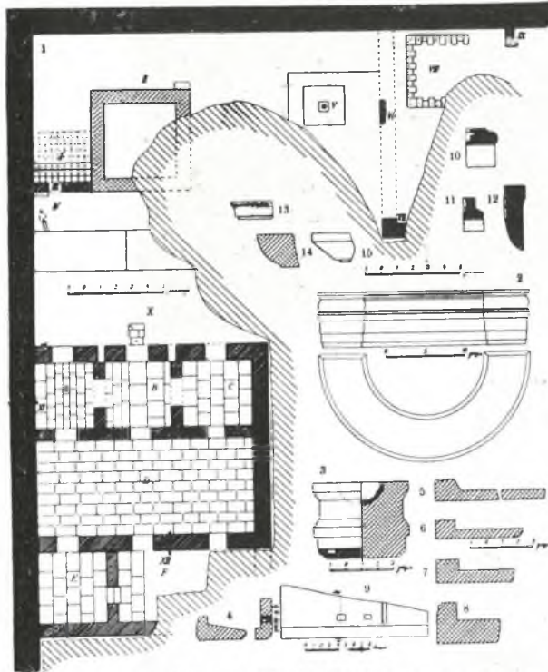
Abb. 225. Plan Škorpil. Nordwestecke des mauerumgrenzten Gebietes. (Aus Aboba-Pliska, Taf. XIV)
