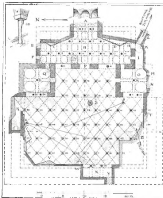
Обр. 190. Планъ на Будрумската „цистерна“ въ Цариградъ споредъ K. Wulzinger
