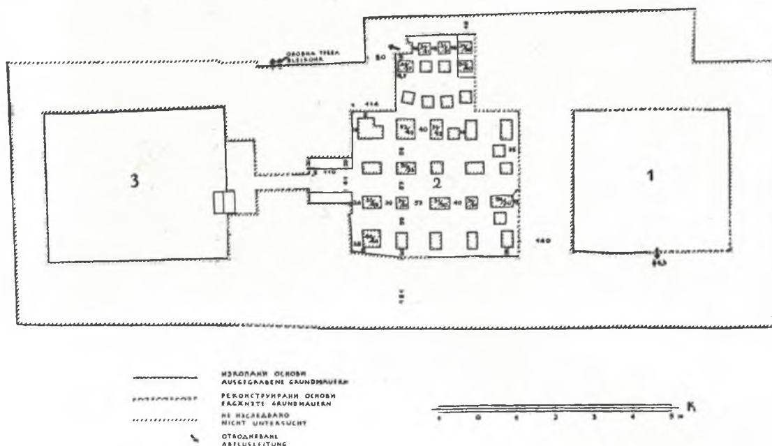
Abb. 222. Gebäude F. Grundriss
