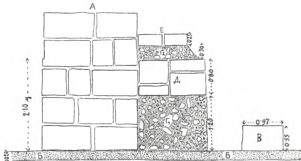
Обр. 187. Разрѣзъ на мѣстото b на обр. 176. А северна стена на Голѣмия дворецъ, Б хоросанена настилка на старъ зидъ ( b ), В запазенъ на мѣсто камъкъ отъ стария зидъ, Г 1 и Г 2 насипъ, Д околень зидъ, Е тротоарна настилка
