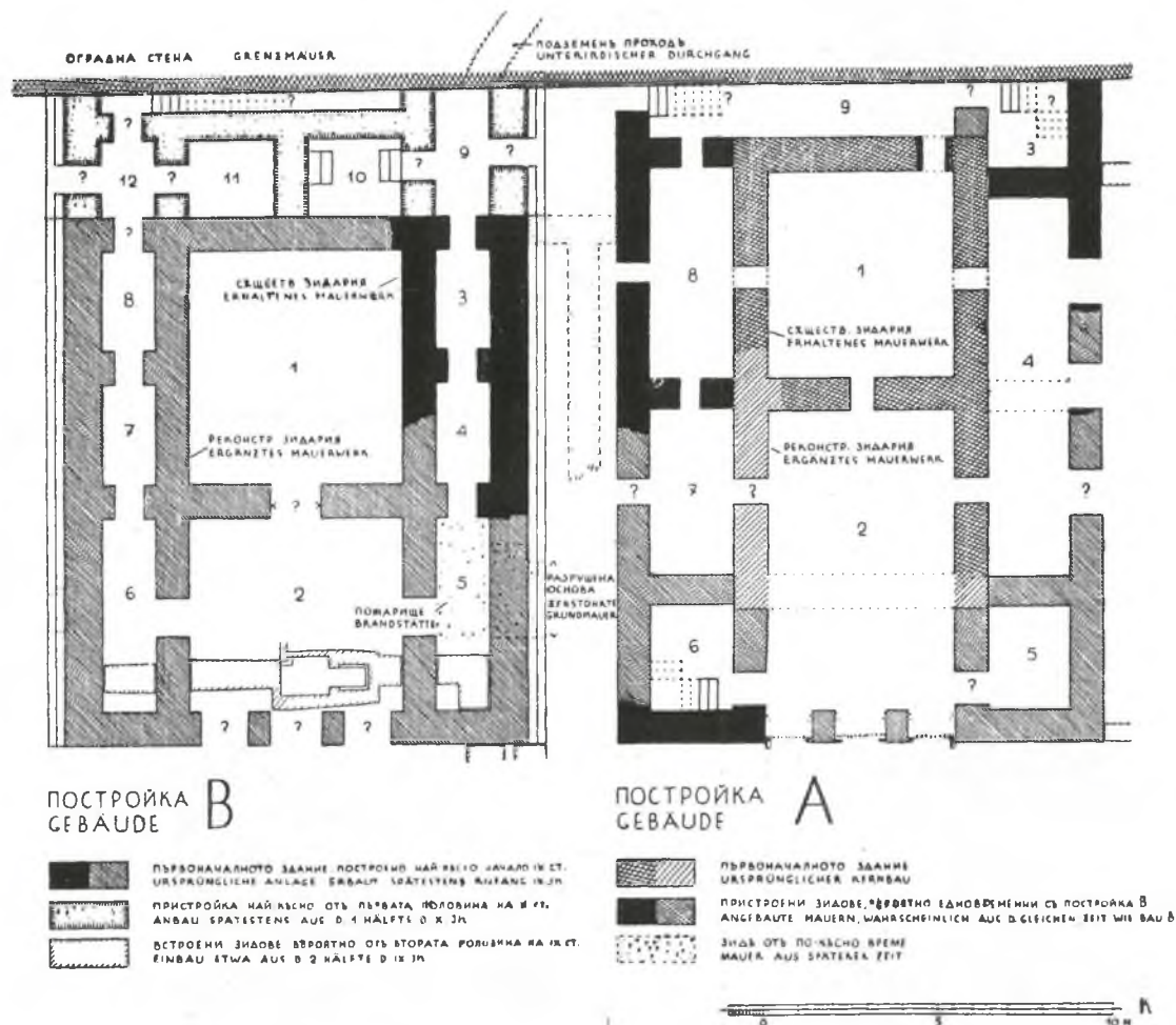
Abb. 193. Gebäude A und B. Neue Aufnahme
