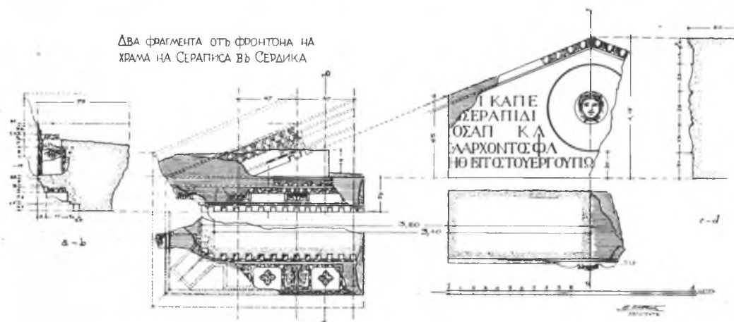
Обр. 314. Свързване на намѣренитѣ фрагменти отъ фронтонa на храма на Сераписа въ София
