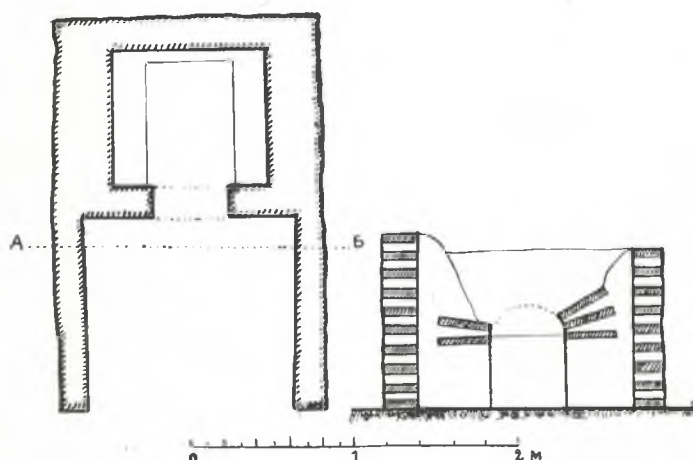
Обр. 169. Планъ и разрѣзъ на пещъта при „Брѣстоветѣ“
