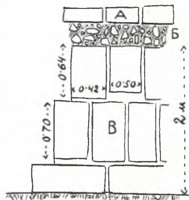
Обр. 182. Разрѣзъ на стена a на помѣщение A
