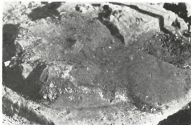
Abb. 215. Gebäude C. Putzrundung an einer Säule
