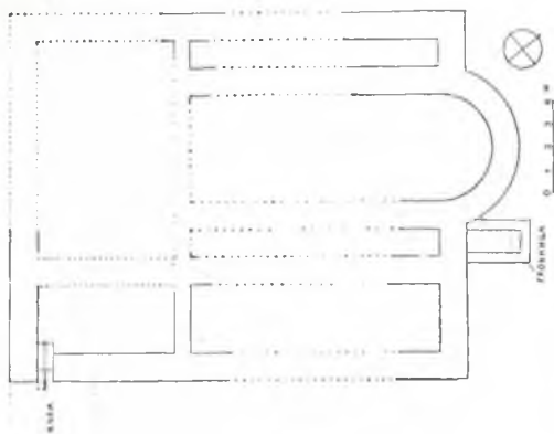
Обр. 385. Планъ на християнска базилика въ Црънча
