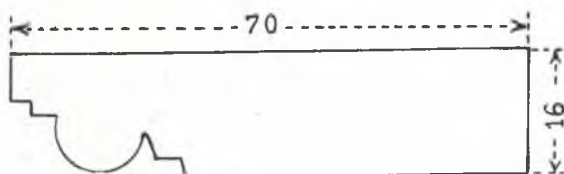
Обр. 167. Профилъ на варовиковъ корнизъ
