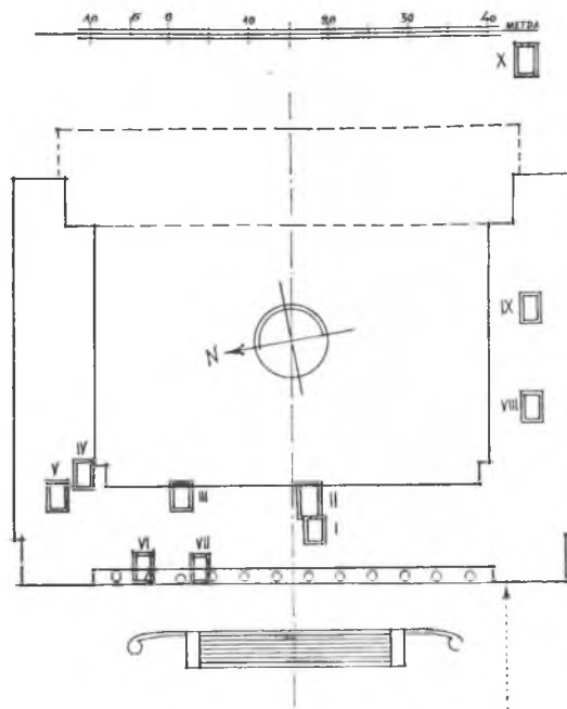
Обр. 334. Ситуационенъ планъ за разположението на открититъ старохристиянски гробници въ основитъ на новостроящата се Народна библиотека въ София
