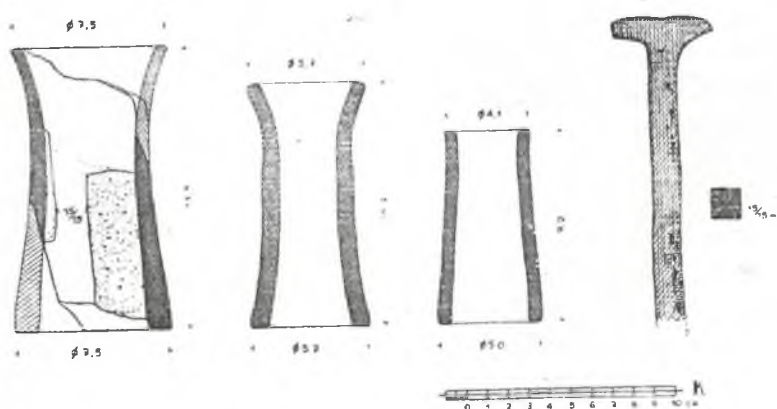
Abb. 205. Tonröhrchen aus den Hypokaustanlagen der Gebäude B und F
