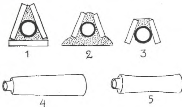
Обр. 163. Разрѣзи на водопроводи и водопроводни трѣби
