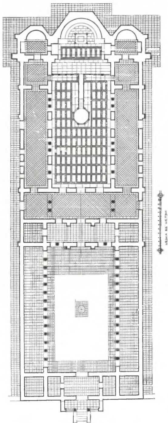
Fig. 162. — La Grande basilique de Pliska (plan Rachénov).
