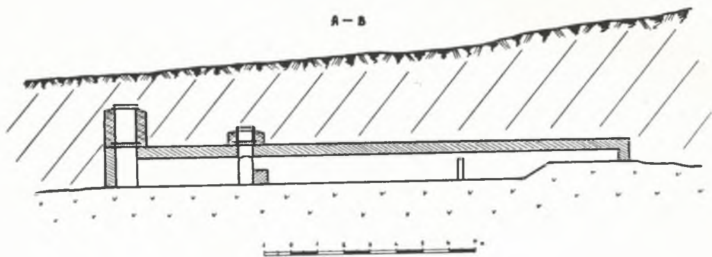
Обр. 153. — Надлъженъ разрѣзъ на римския каптажъ на старозагорскитѣ бани. Fig. 153. — Coupe longitudinale du captage romain des sources thermales près de Stara-Zagora.
