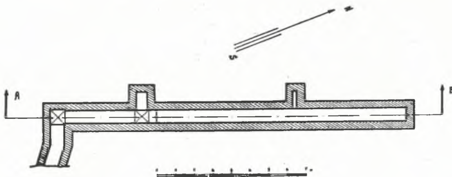
Обр. 155. — Планъ на римския каптажъ на старозагорскитѣ бани. Fig. 155. — Plan du captage romain des sources thermales près de Stara-Zagora.
