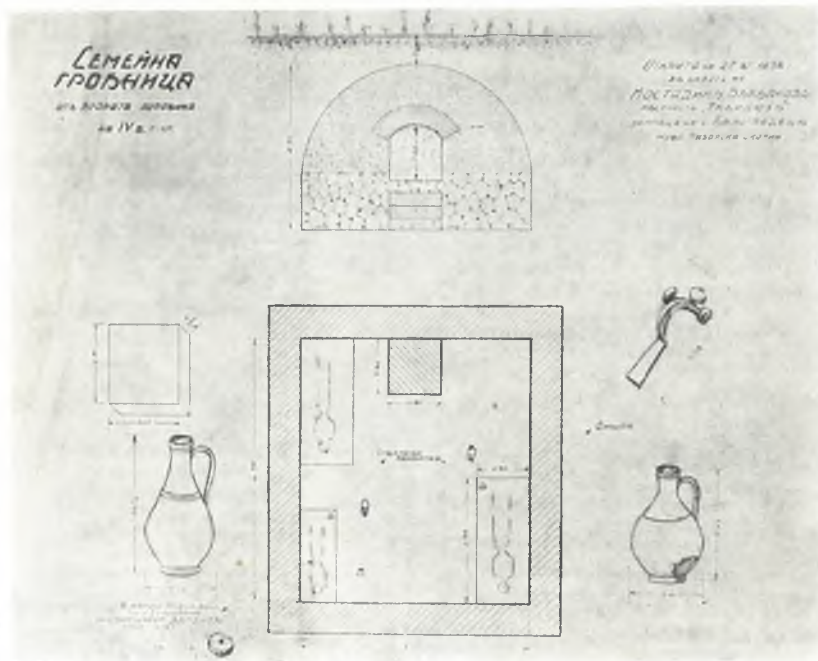
Обр. 209. — Късноримска гробница при с. Бѣлоградещъ. Fig. 209. — Tombeau romain près de Bélogradetz.
