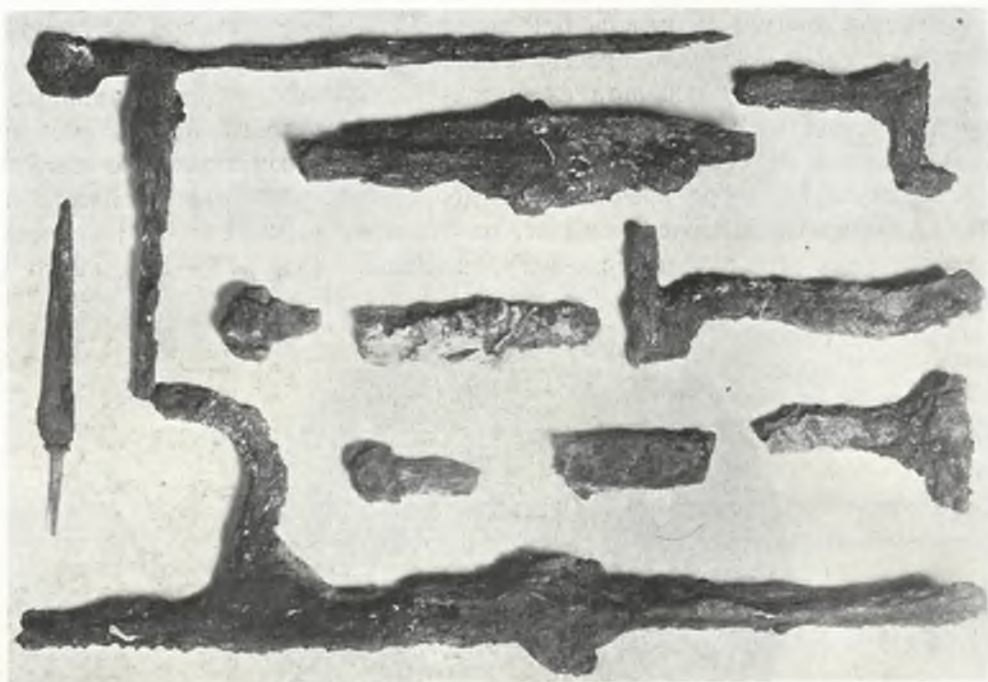
Обр. 76. — Части отъ желѣзенъ сгъваемъ столъ. Abb. 76. — Bruchstücke eines eisernen Klappstuhles.
